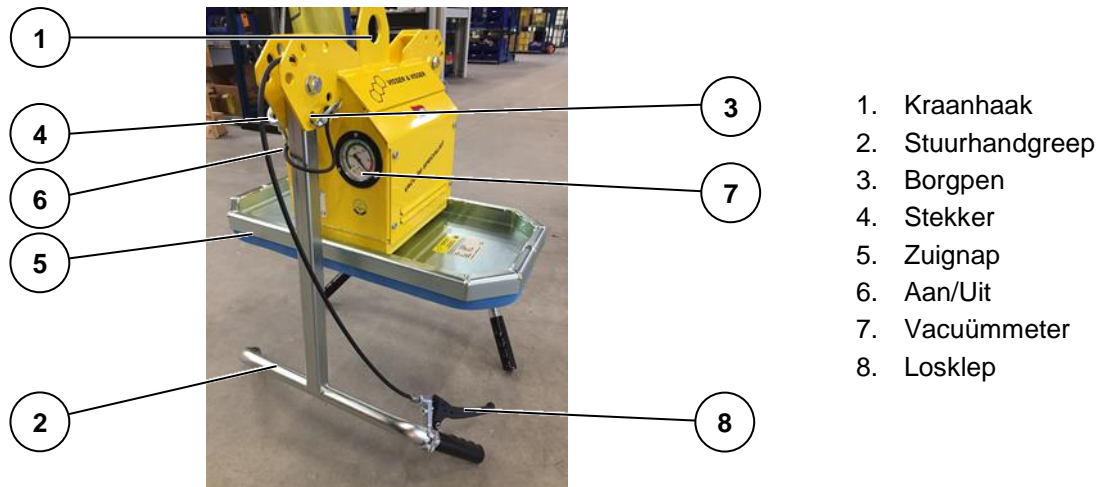
Figuur 2: Hoofdonderdelen van de machine
