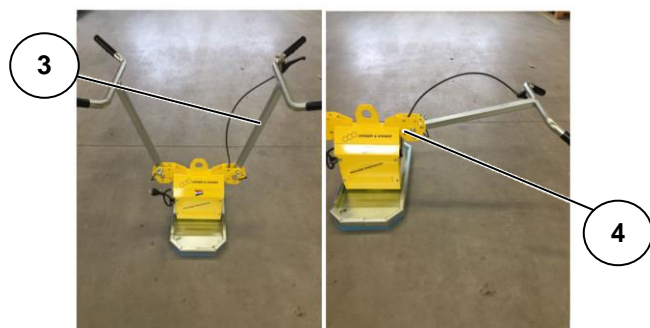
Figuur 8: Werkstand
