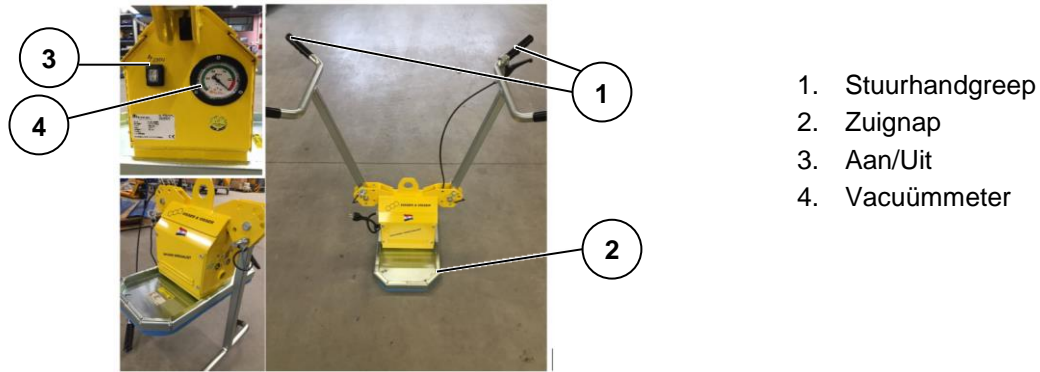
Figuur 1: Werkingsprincipe
