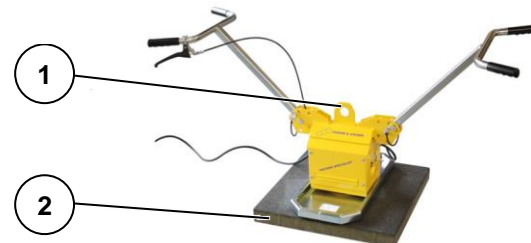
Figuur 10: Aan machine bevestigen (voorbeeld)
