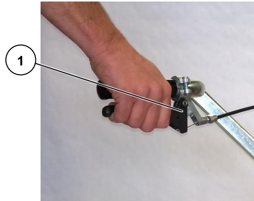
Figuur 13: Losklep
